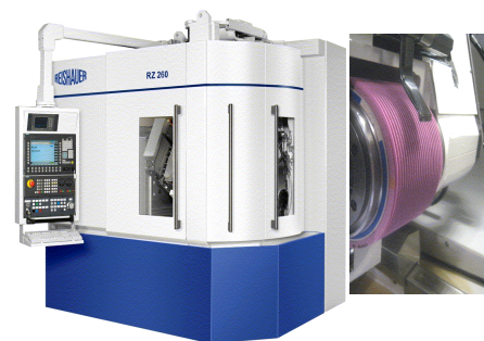
Wälzschleifen: Reishauer RZ 260
